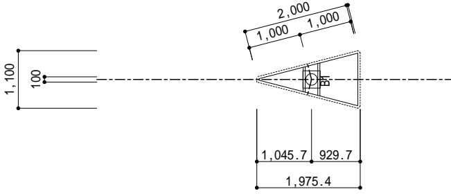
上部平面図 1/100
